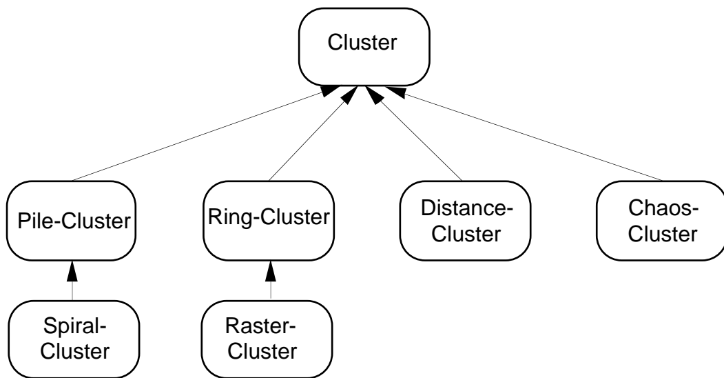
Abbildung 3.16: Typen von sog. „Clustern“ zur Anordnung von Fenstern. Die Abbildung wurde aus [Herczeg 86] übernommen.
