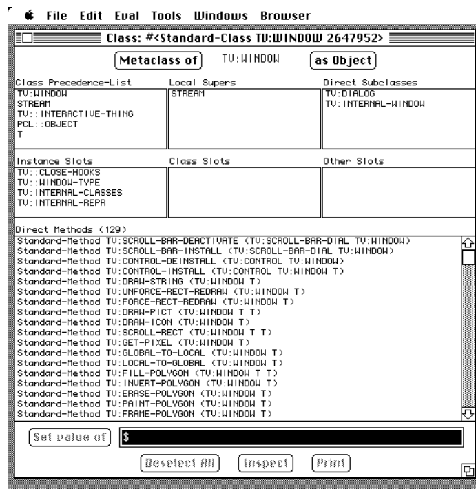
Abbildung 3.7: CLOS-Klasseninspektor-Dialog. Die Tabelle für die Methoden der gezeigten Klasse wird bei vergrößerter Darstellungsfläche auch entsprechend vergrößert. Die oberen Tabellen benötigen nicht mehr Raum.
