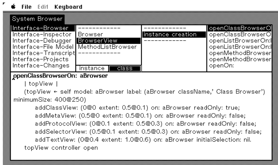
Abbildung 3.17: Systeminspektor der Programmierungsumgebung Smalltalk-80. Gezeigt wird der Quelltext einer Methode zur Erzeugung eines Klasseninspektors.
