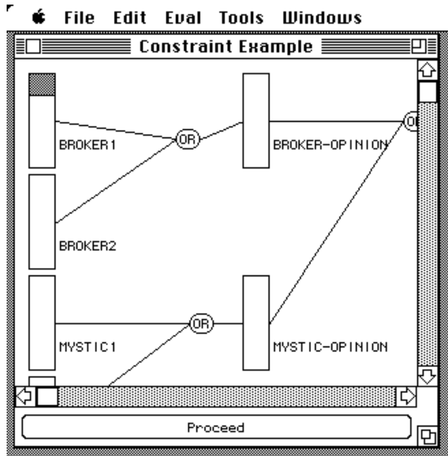
Abbildung 5.5: Einschränkungnetz mit Schaltfläche zur Überwachung der Propagation.
