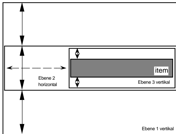
Abbildung 3.9: Schematische Darstellung von geschachtelten Boxen. Pfeile stellen Füllangaben dar. Füllangaben der Ebene 1 sind unabhängig von denen der Ebene 3.
