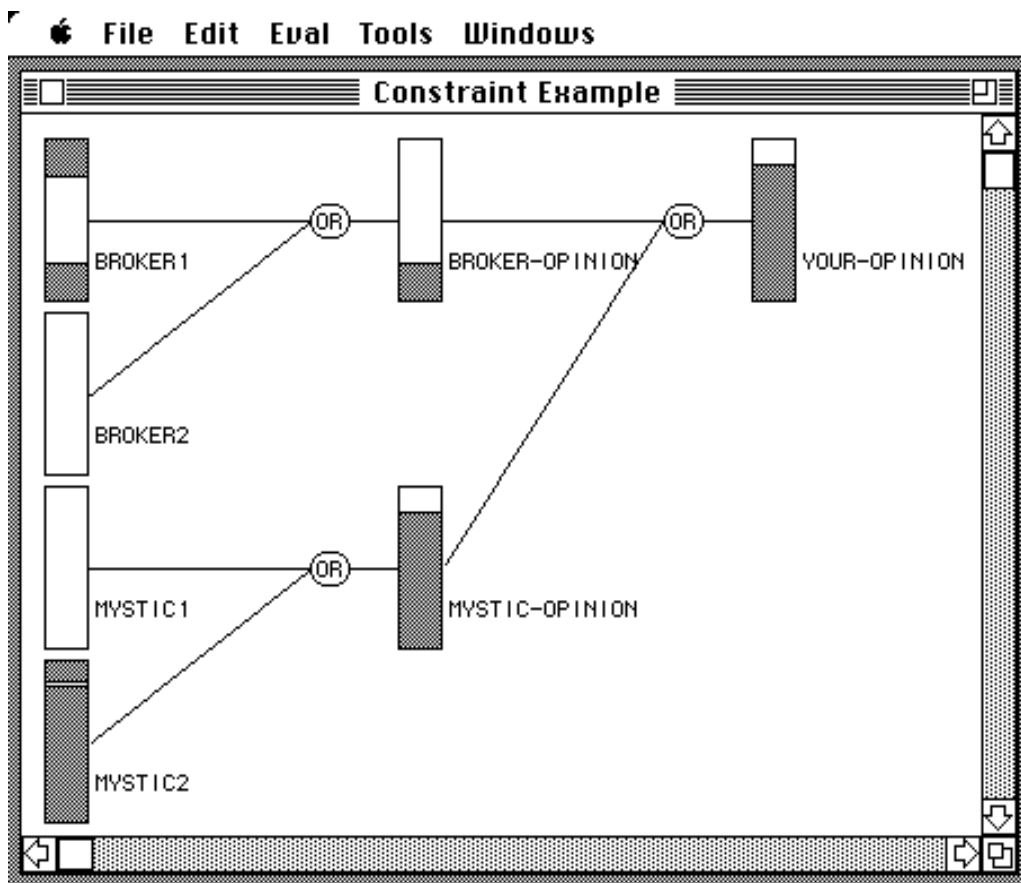
Abbildung 5.4: Zustand des Einschränkungsnetzes nach der Propagation.
