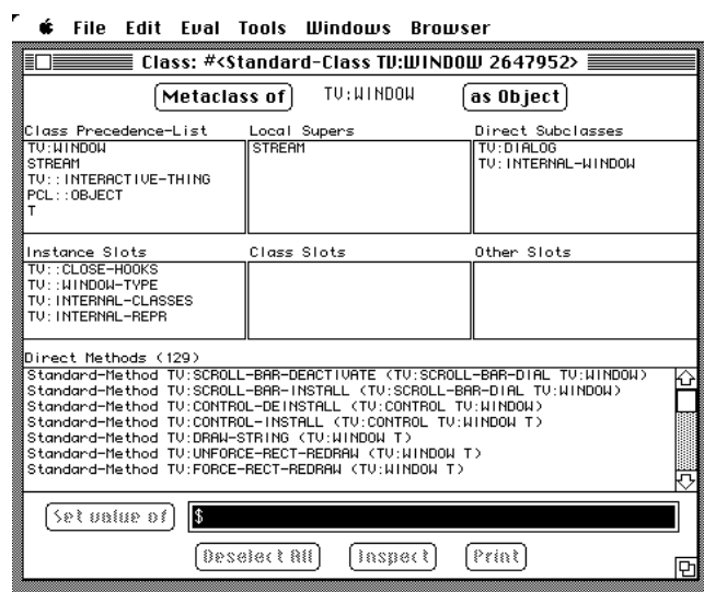
Abbildung 3.6: CLOS-Klasseninspektor-Dialog.
