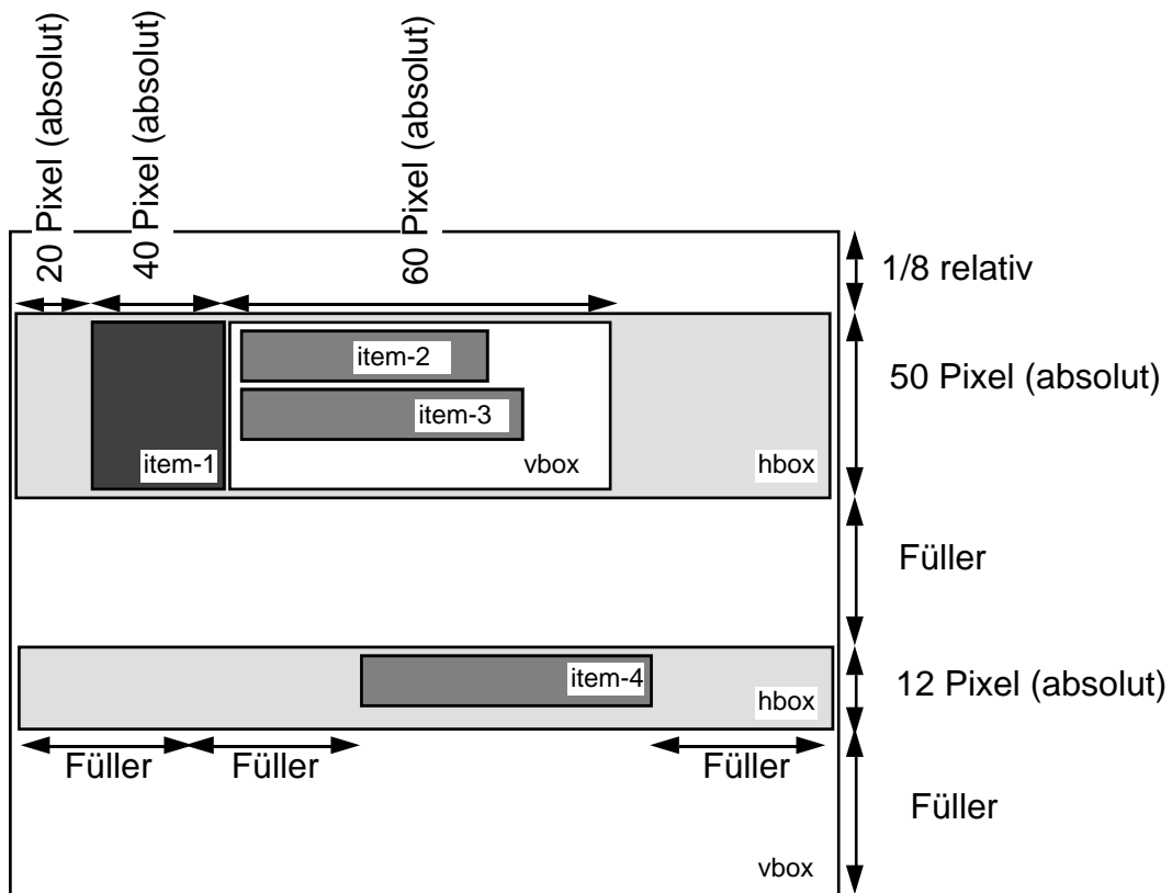
Abbildung 3.5: Verwendung einer :fbox.
