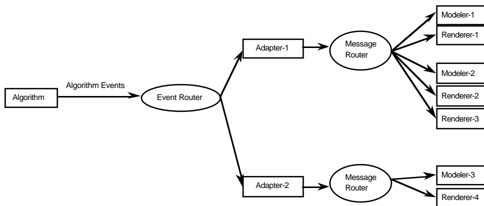
Abbildung 4.4: Verteilungsschema für „Algorithmenergebnisse“ (nach [Brown 88]).
