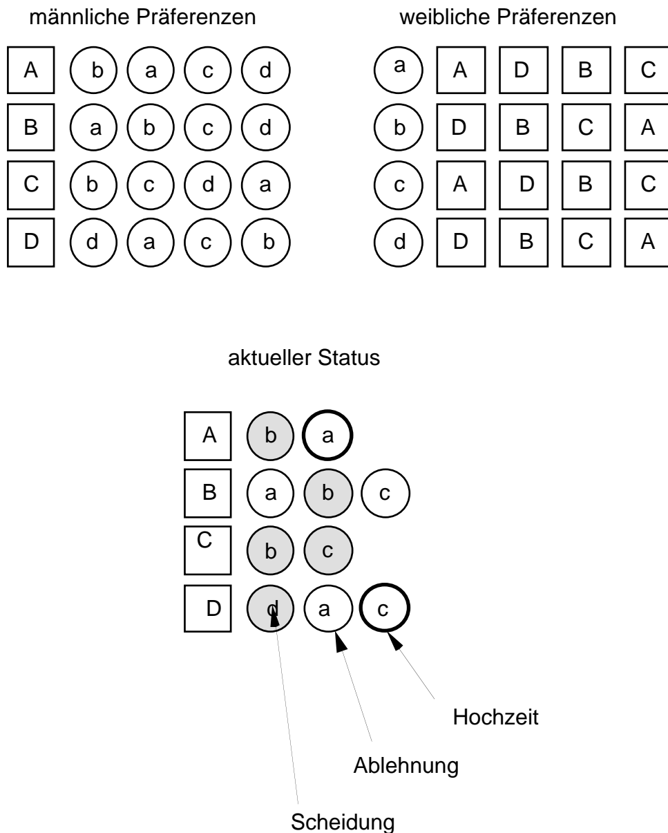
Abbildung 6.1: Schnappschuß der Zuordnung im Algorithmus „Stabile Heirat“ (nach [Hsia & Ambler 88]).
