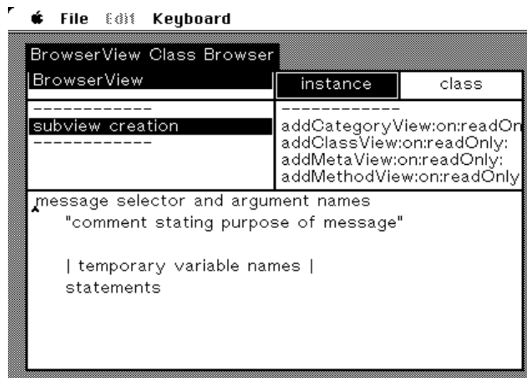
Abbildung 3.18: Klasseninspektor für die Klasse BrowserView.
