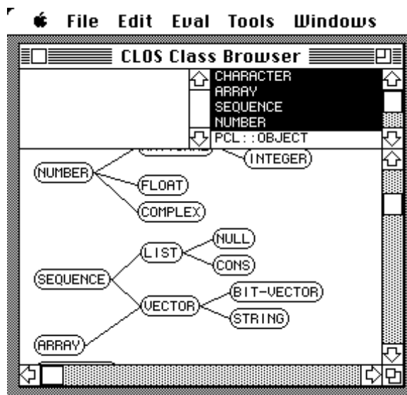
Abbildung 3.15: Ein Ausschnitt aus der CLOS-Klassenhierarchie.
