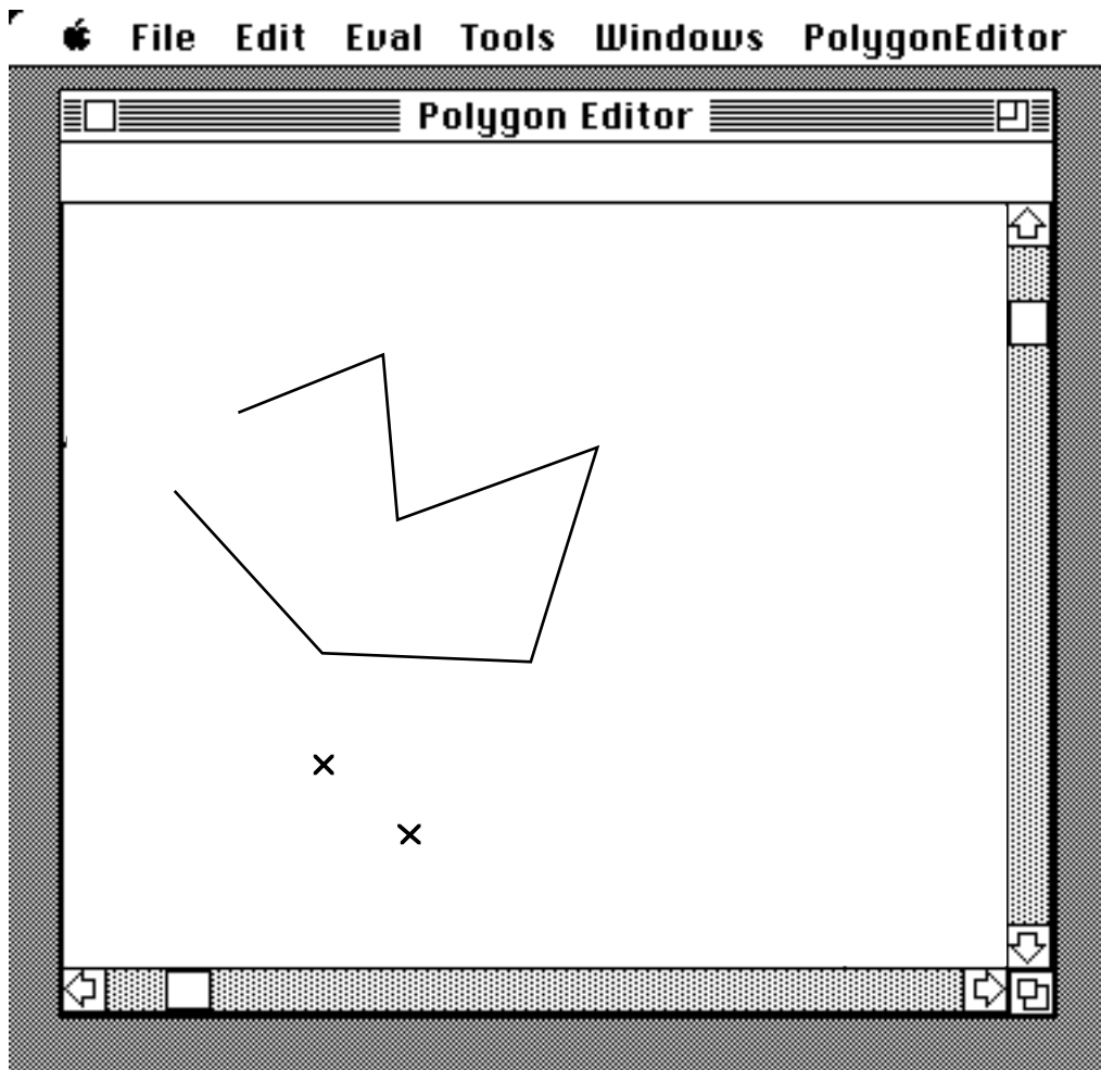
Abbildung 3.2: Ein Polygoneditor-Dialog.
