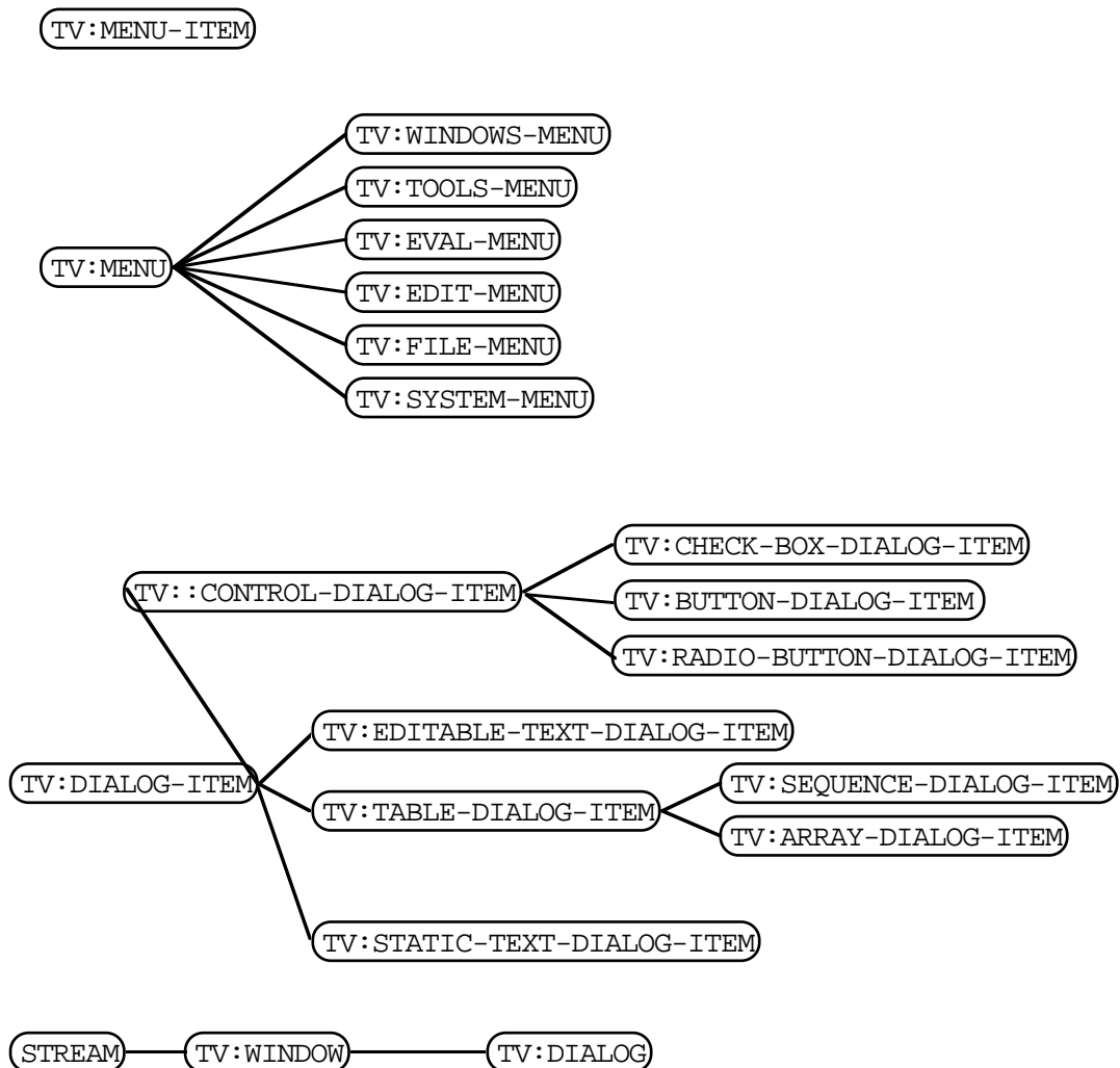
Abbildung 3.1: Ausschnitt aus der Klassenhierarchie. Enthalten sind die CLOS-Klassen, die für von der „Allegro“-Umgebung übernommene ObjectLisp-Klassen stehen.
