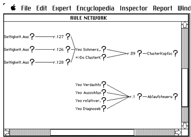
Abbildung 2.3: Darstellung eines Regelnetzwerks in Nextperts.
