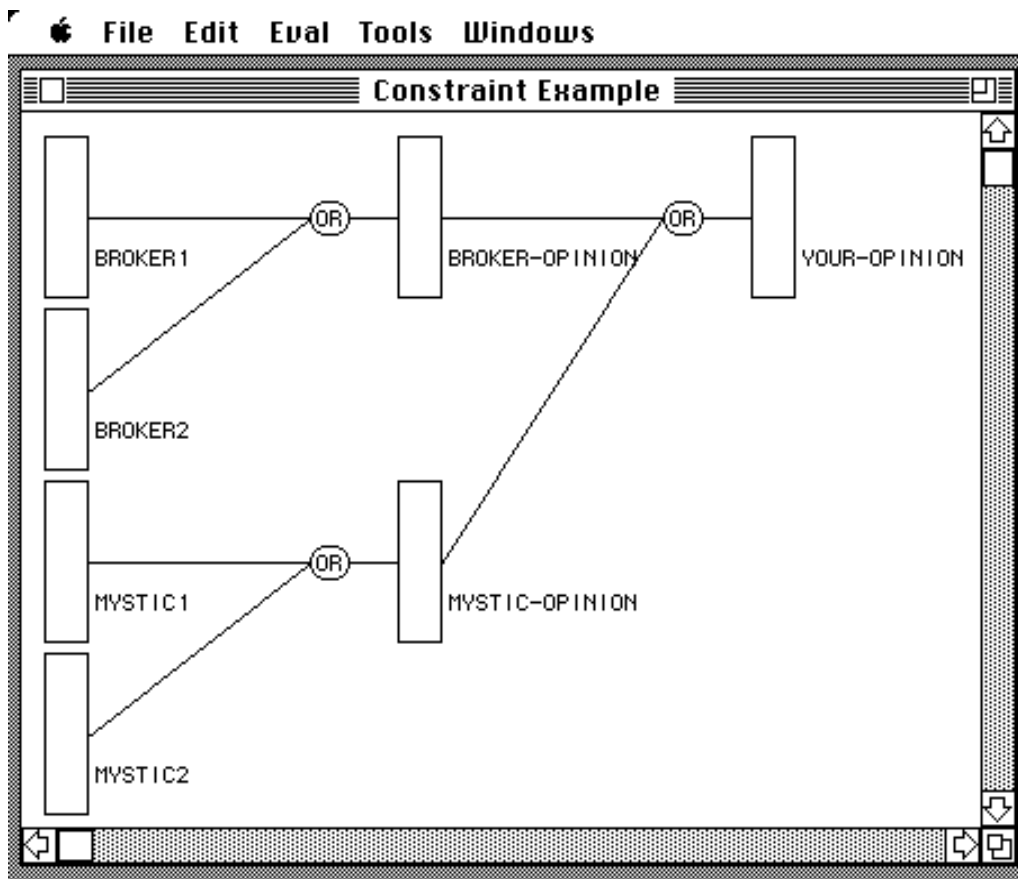
Abbildung 5.3: Einschränkungnetz dargestellt als DAG.
